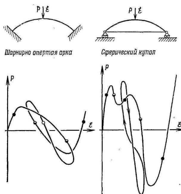
Рис. 1 – Последовательные складки на траекториях равновесия пологой арки и сферического купола
